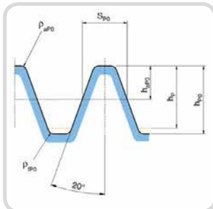
Bezugsprofil I / Für Fertigbearbeitung Basic Rack Profile I / For finishing
