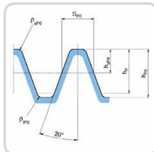
Bezugsprofil II / Für Fertigbearbeitung Basic Rack Profile II / For finishing
