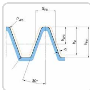
Bezugsprofil IV / Für Vorbereitung zum Schlichten Basic Rack Profile IV / Preshaping for finishing
