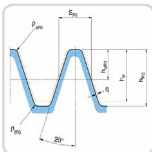
Bezugsprofil III / Für Vorbereitung zum Schleifen oder Schaben Basic Rack Profile III / Preshaping for grinding or shaving
